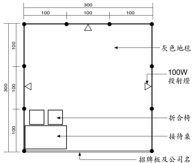
標準攤位平面圖
